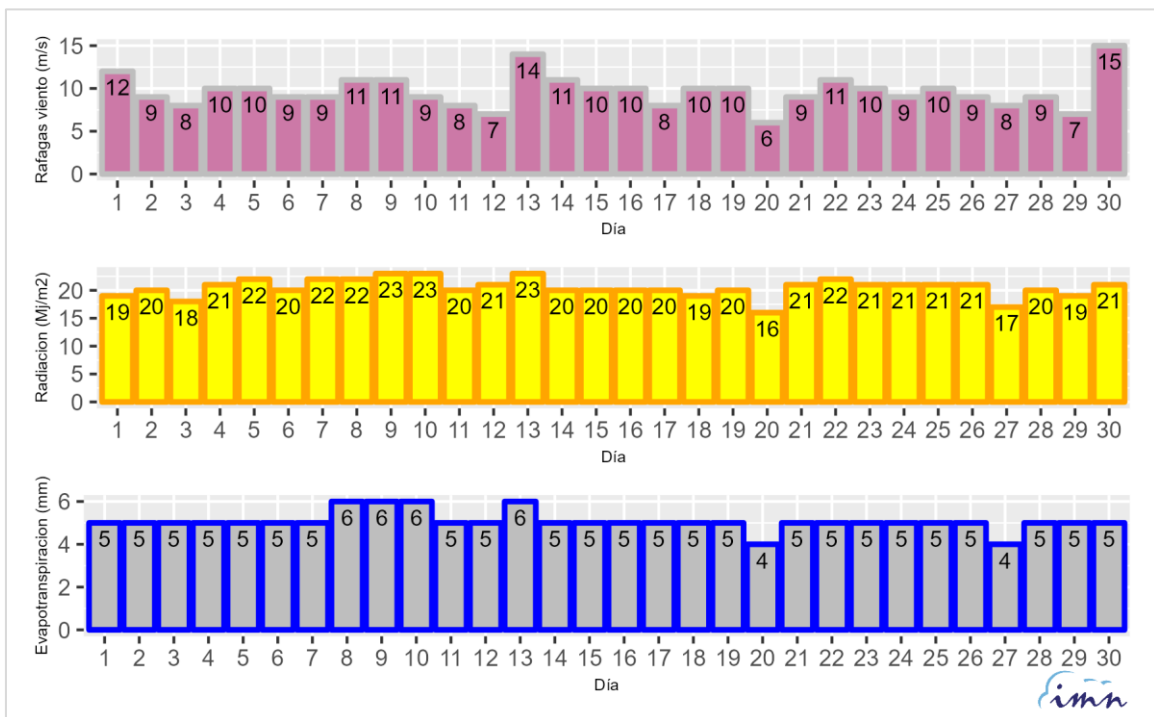
Figura 4.b. Promedio diario de viento máximo (m/s), radiación solar (MJ/m²) y evapotranspiración referencia (mm) para junio 2024 en la región cañera Región Norte .
