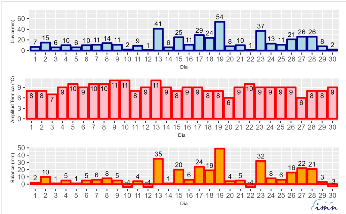
Figura 4.a. Promedio diario de precipitación (mm), amplitud térmica (°C), balance hídrico (mm) para junio 2024 en la región cañera Región Norte .
