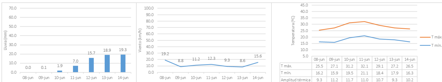
Figura 10. Pronóstico de precipitación (mm), viento (km/h) y temperatura (°C) para el periodo del 08 de junio al 14 de junio en la región cañera Zona Sur.
