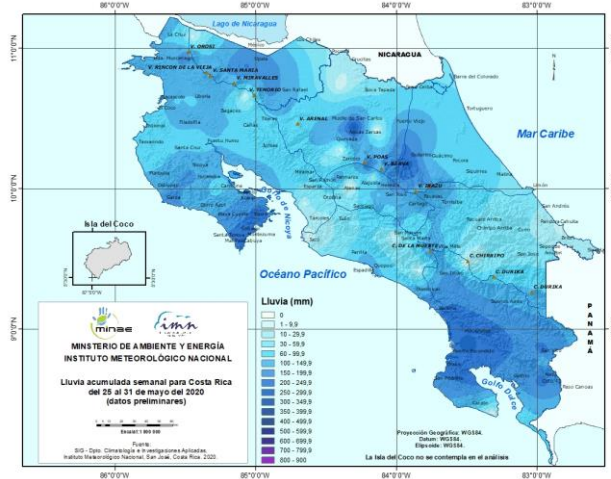
Figura 1. Valores acumulados de la precipitación (mm) durante la semana del 25 de mayo al 31 de mayo del 2020 (datos preliminares).
