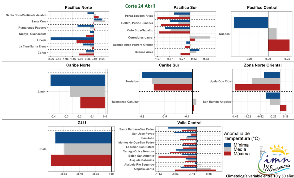
Figura 1. Anomalías de temperatura del 1-24 abril del 2023, respecto al periodo climatológico variable de entre 10 y 30 años, para las diferentes regiones climáticas del país. Donde la temperatura máxima se aprecia en color rojo, la temperatura mínima en color azul y la temperatura media en gris. (Fuente: Rosangelica Montero Acuña, UCLIM-IMN)
