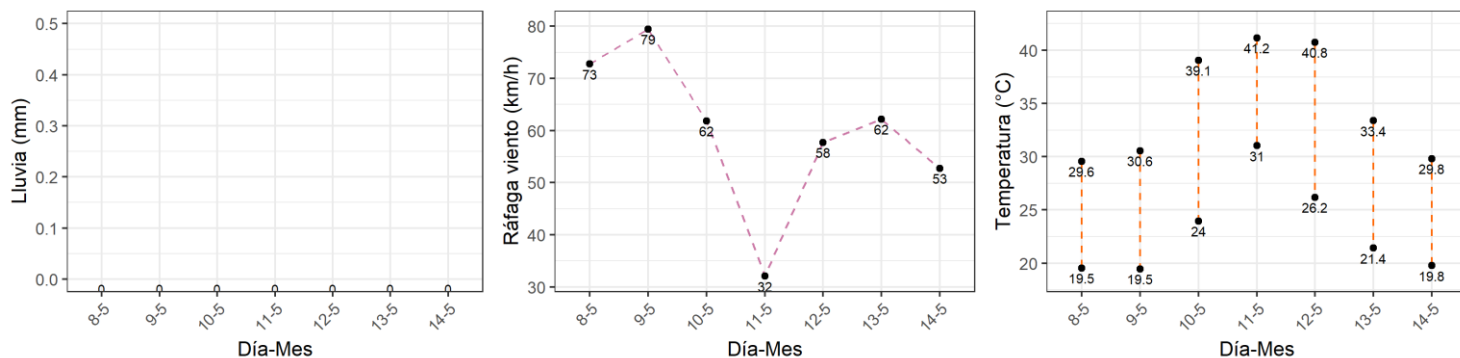
Figura 2. Pronóstico de precipitación (mm), viento (km/h) y temperatura (°C) del 08 al 14 de mayo en la región cañera Guanacaste Este.
