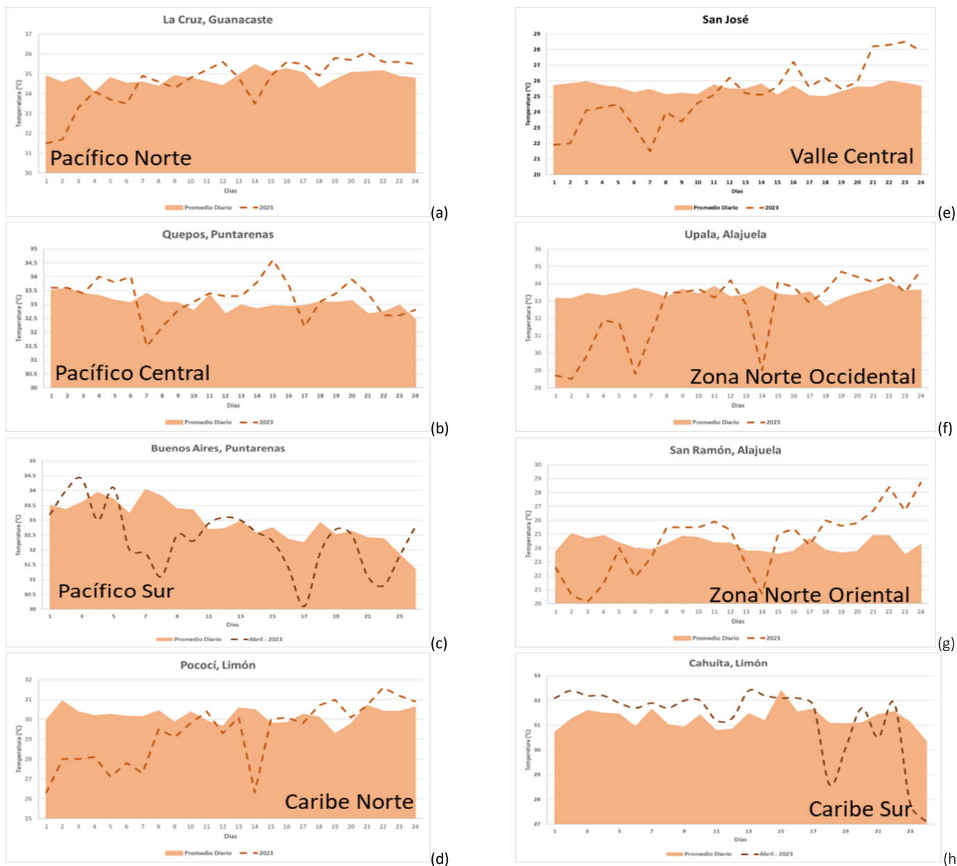
Figura 2. Gráficos de temperatura máxima diaria del 1-24 de abril del 2023 para las regiones climáticas del (a) Pacífico Norte, (b) Pacífico Central, (c) Pacífico Sur, (d) Caribe Norte, (e) Valle Central, (f) Zona Norte Occidental, (g) Zona Norte Oriental y (h) Caribe Sur. Se muestra promedio histórico en contorno naranja y valores del 2023 en línea punteada roja. (Fuente: Rosangelica Montero Acuña y Karina Hernández Espinoza; UCLIM-IMN).
