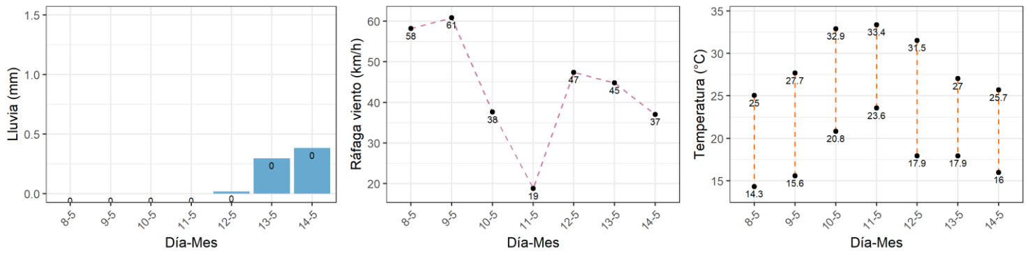
Figura 6. Pronóstico de precipitación (mm), viento (km/h) y temperatura (°C) del 08 al 14 de mayo en la región cañera Valle Central (Este y Oeste).
