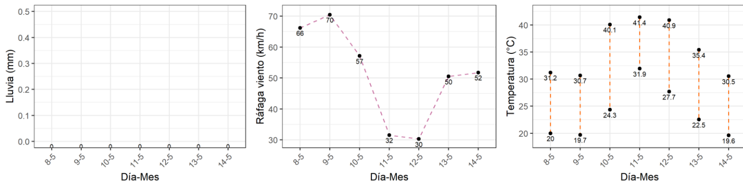
Figura 3. Pronóstico de precipitación (mm), viento (km/h) y temperatura (°C) del 08 al 14 de mayo en la región cañera Guanacaste Oeste.
