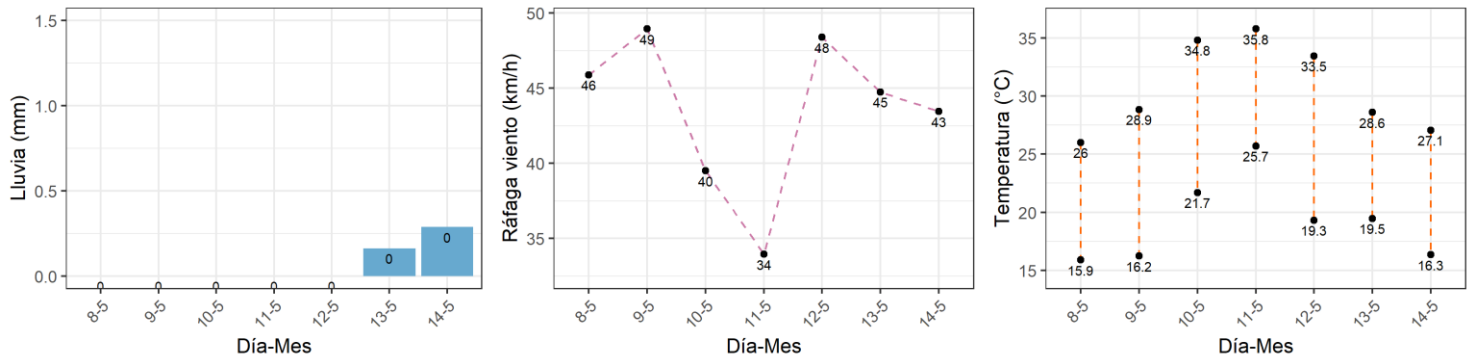
Figura 5. Pronóstico de precipitación (mm), viento (km/h) y temperatura (°C) del 08 al 14 de mayo en la región cañera Región Norte.
