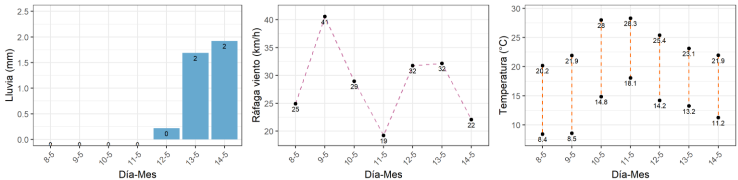
Figura 7. Pronóstico de precipitación (mm), viento (km/h) y temperatura (°C) del 08 al 14 de mayo en la región cañera Turrialba (Alta y Baja).
