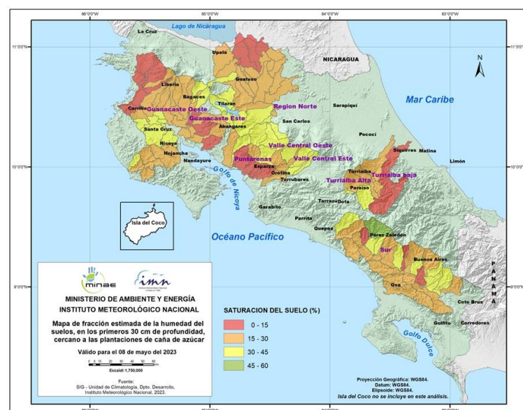
Figura 09. Mapa de fracción estimada de la humedad en porcentaje (%), en los primeros 30 cm de profundidad, cercano a las plantaciones de caña de azúcar, válido para el 08 de mayo de 2023.
