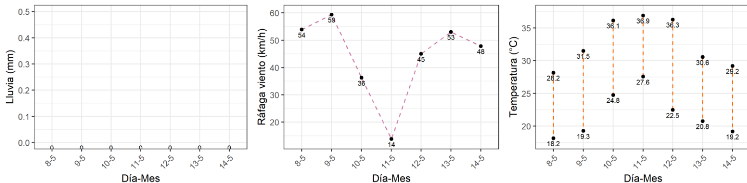
Figura 4. Pronóstico de precipitación (mm), viento (km/h) y temperatura (°C) del 08 al 14 de mayo en la región cañera Puntarenas.
