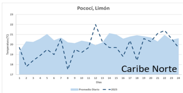
Figura 3. Gráficos de temperatura mínima diaria del 1-24 de abril del 2023 para las regiones climáticas del (a) Pacífico Norte, (b) Pacífico Central, (c) Pacífico Sur, (d) Caribe Norte, (e) Valle Central, (f) Zona Norte Occidental, (g) Zona Norte Oriental y (h) Caribe Sur. Se muestra el promedio histórico en contorno celeste y valores del 2023 en línea punteada azul. (Fuente: Rosangelica Montero Acuña y Karina Hernández Espinoza; UCLIM-IMN).
