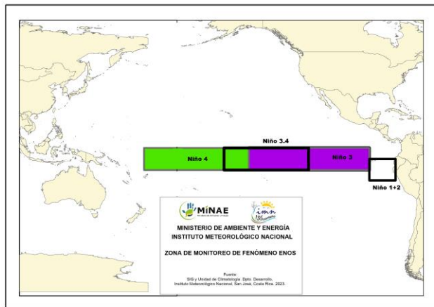
Figura 4. Regiones de monitoreo del fenómeno El Niño Oscilación del Sur (ENOS). (Fuente: UCLIM-IMN)
