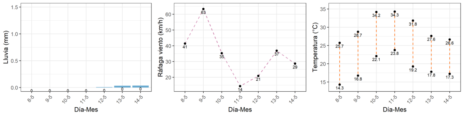
Figura 8. Pronóstico de precipitación (mm), viento (km/h) y temperatura (°C) del 08 al 14 de mayo en la región cañera Región Sur.
