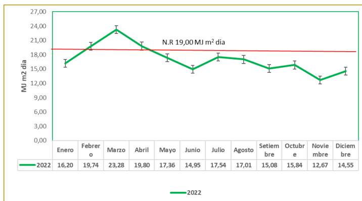
Figura 2. Radiación solar ( \text{MJ m}^2 \text{ día} ), ocurrida en el año 2022. Estación meteorológica finca el Cántaro, Cañas, Guanacaste.
