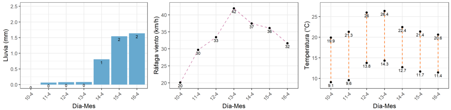
Figura 7. Pronóstico de precipitación (mm), viento (km/h) y temperatura (°C) del 10 al 16 de abril en la región cañera Turrialba (Alta y Baja).
