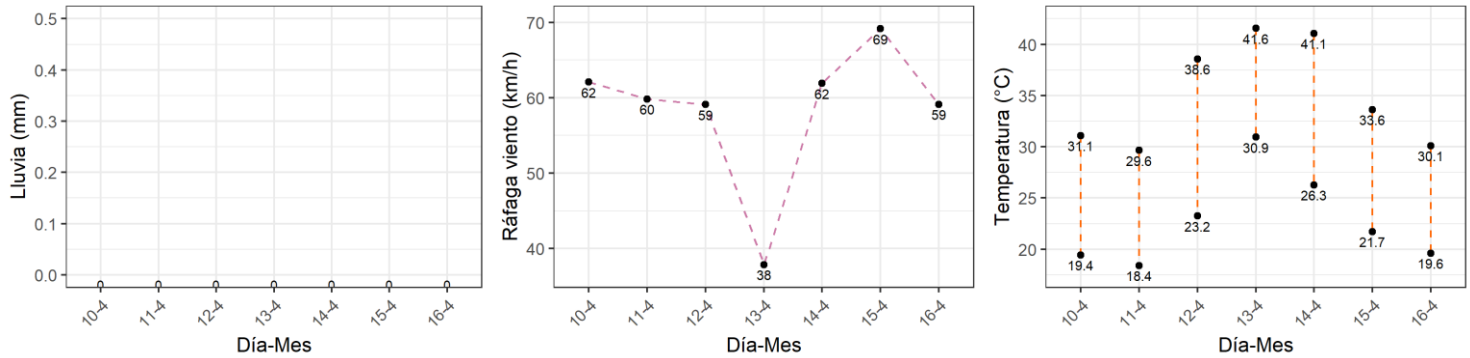
Figura 3 Pronóstico de precipitación (mm), viento (km/h) y temperatura (°C) del 10 al 16 de abril en la región cañera Guanacaste Oeste.
