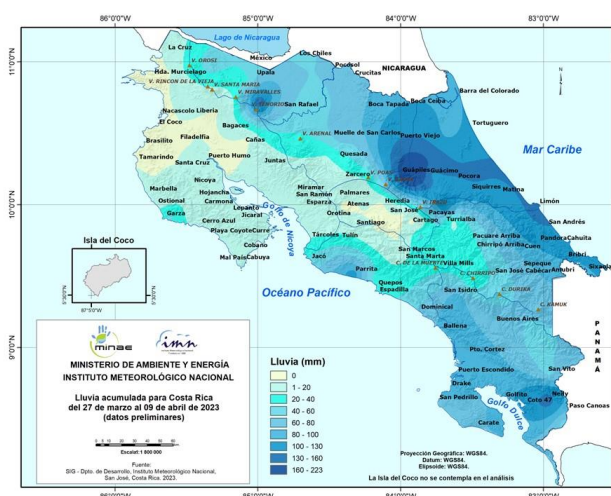
Figura 1. Valores acumulados de la precipitación (mm) durante la quincena del 27 de marzo al 09 de abril del 2023.
