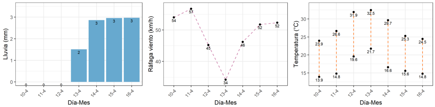
Figura 6. Pronóstico de precipitación (mm), viento (km/h) y temperatura (°C) del 10 al 16 de abril en la región cañera Valle Central (Este y Oeste).
