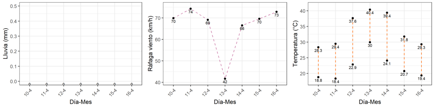
Figura 2. Pronóstico de precipitación (mm), viento (km/h) y temperatura (°C) del 10 al 16 de abril en la región cañera Guanacaste Este.
