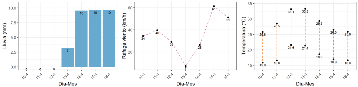
Figura 8. Pronóstico de precipitación (mm), viento (km/h) y temperatura (°C) del 10 al 16 de abril en la región cañera Región Sur.
