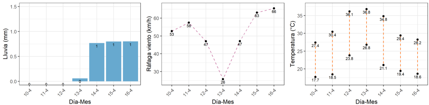
Figura 4. Pronóstico de precipitación (mm), viento (km/h) y temperatura (°C) del 10 al 16 de abril en la región cañera Puntarenas.
