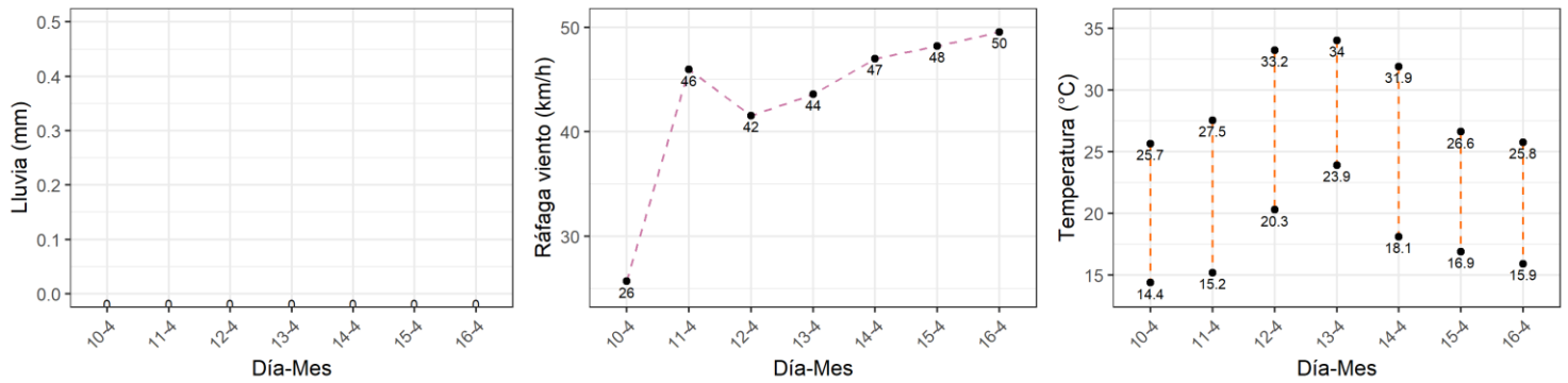
Figura 5. Pronóstico de precipitación (mm), viento (km/h) y temperatura (°C) del 10 al 16 de abril en la región cañera Región Norte.
