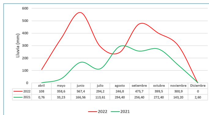
Figura 1. Precipitación mensual (mm) para los periodos 2021 y 2022. Datos tomados de la estación meteorológica Ingenio Taboga, Cañas, Guanacaste.
