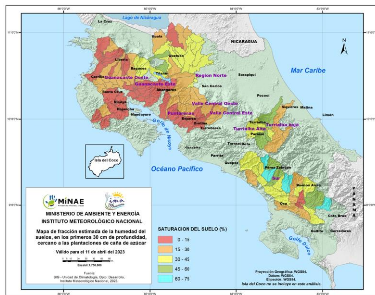
Figura 09. Mapa de fracción estimada de la humedad en porcentaje (%), en los primeros 30 cm de profundidad, cercano a las plantaciones de caña de azúcar, válido para el 11 de abril de 2023.
