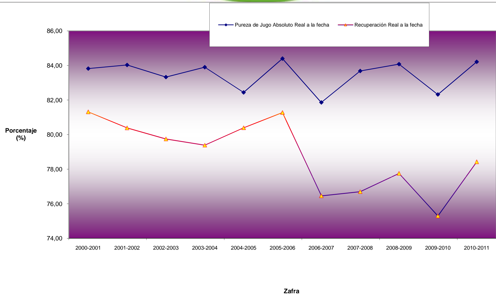
Figura 2: Comparativo de Pureza de Jugo Absoluto Real a la fecha contra la recuperación real a la fecha del último día de zafra desde la zafra 2000-2001 a la zafra 2010-2011. (Fuente: Reporte de Producción Ingenio Taboga S.A.)
