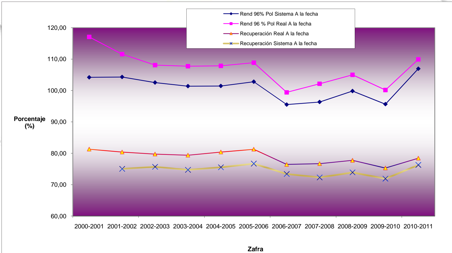
Figura 1: Comparativo de Rendimientos 96% Pol real y del sistema, a la fecha del último día de zafra y comparativo de Recuperación real y del sistema, a la fecha del último día de zafra. Se incluyen los datos desde la zafra 2000-2001 a la zafra 2010-
