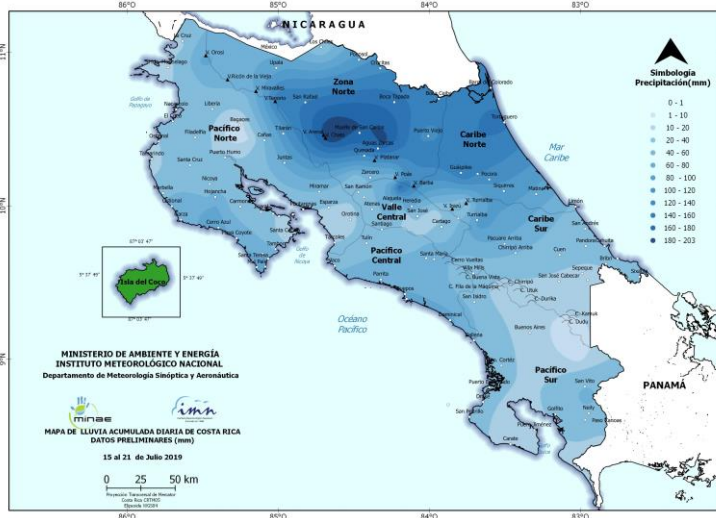
Figura 1. Valores acumulados de la precipitación (mm) durante la semana de 15 al 21 de julio (generado utilizando datos preliminares).
