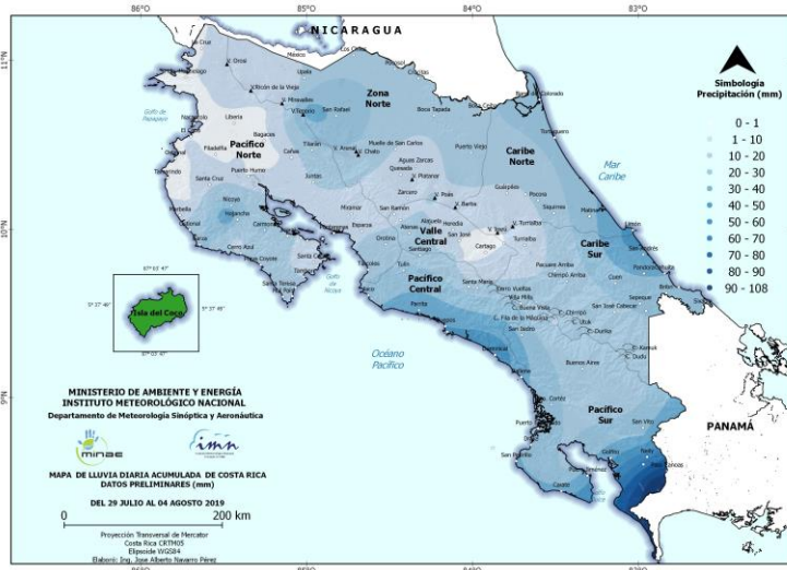
Figura 1. Valores acumulados de la precipitación (mm) durante la semana de 29 de julio al 4 de agosto (generado utilizando datos preliminares).
